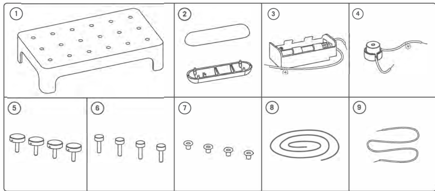
Деталь 1. Платформа, Деталь 2. Ручка, Деталь 3. Корпус батарейного відсіку, Деталь 4. Електричний зумер, Деталь 5. Великі штифти x 4, Деталь 6. Маленькі штифти x 4, Деталь 7: Металеві контакти x 4, Деталь 8. Дріт, Деталь 9: Ізольований дріт. Також необхідні, але не входять в комплект: 2 батареї AAA 1,5В та ножиці для відрізання дротів.
